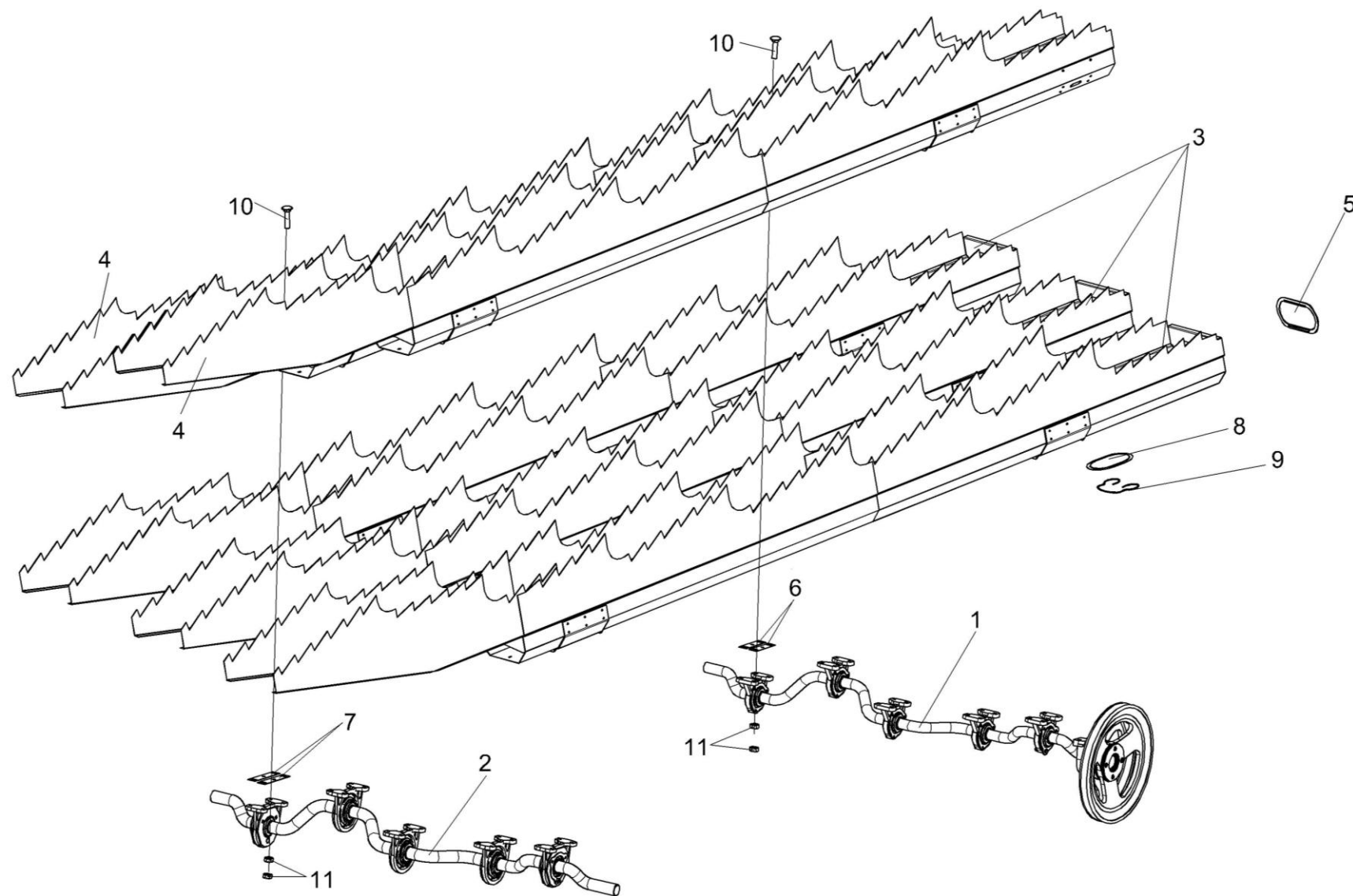
Рисунок 67 – Соломотряс КЗК-12-0212040
