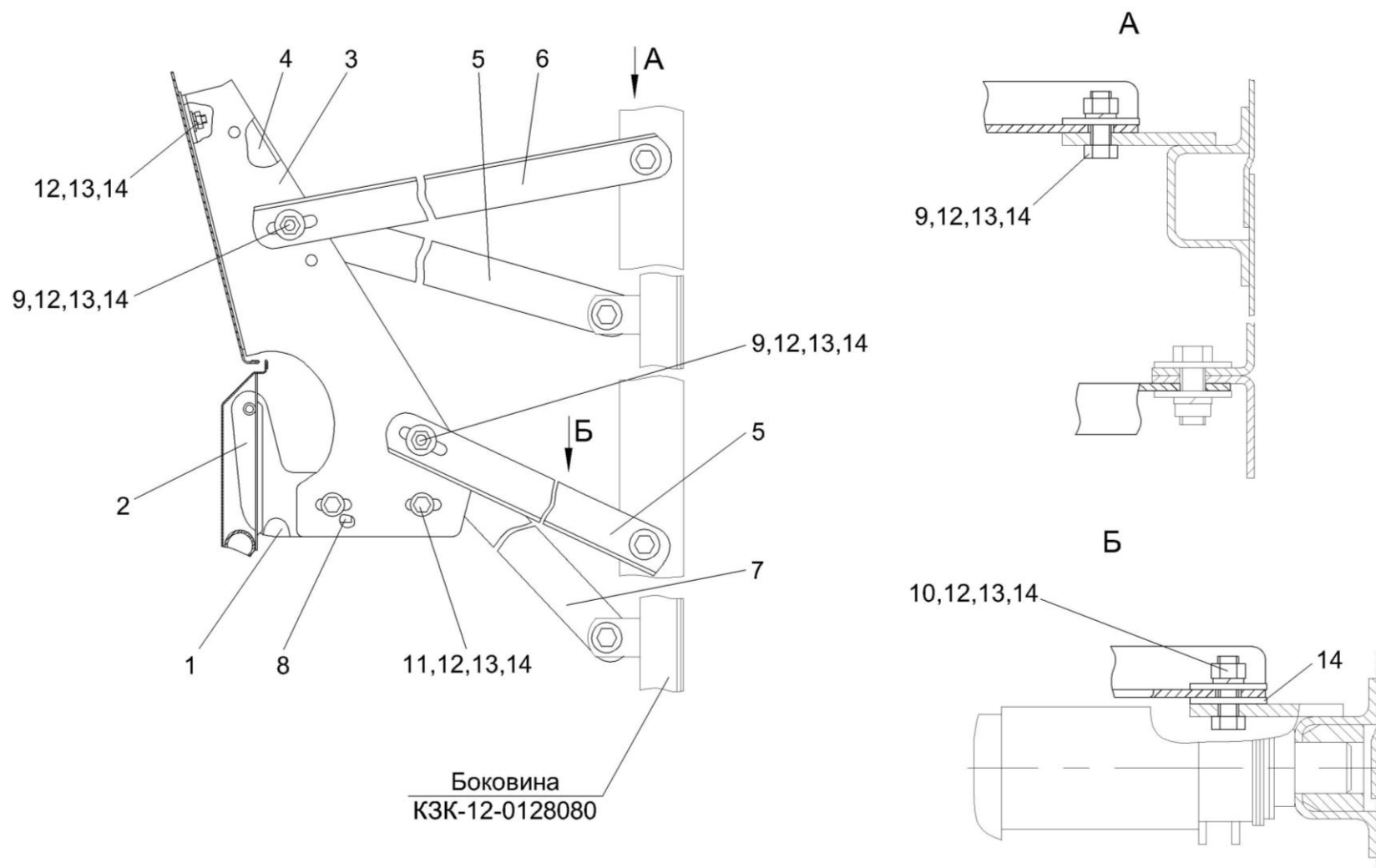
Рисунок 182 – Установка кронштейна КЗК 0128420-01
