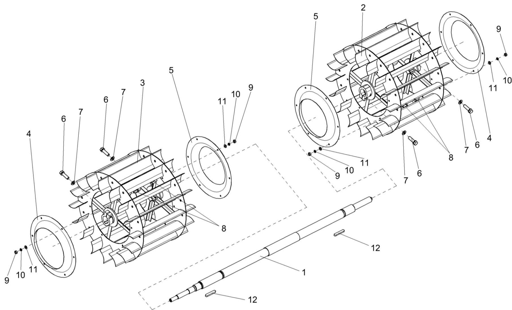
Рисунок 93 – Крылач КЗК-10-0217010
