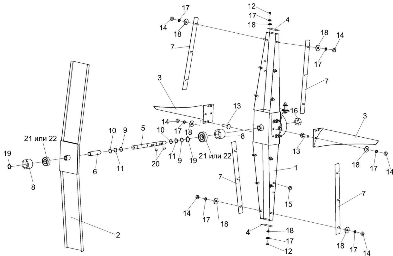
Рисунок 206 – Пылесъемник КЗК-12-3-0112130А
