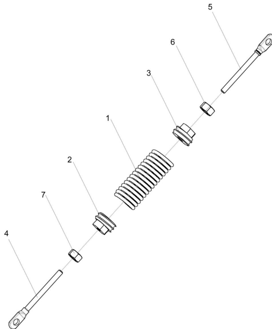
Рисунок 218 – Пружина КЗК-12-3-0220050
