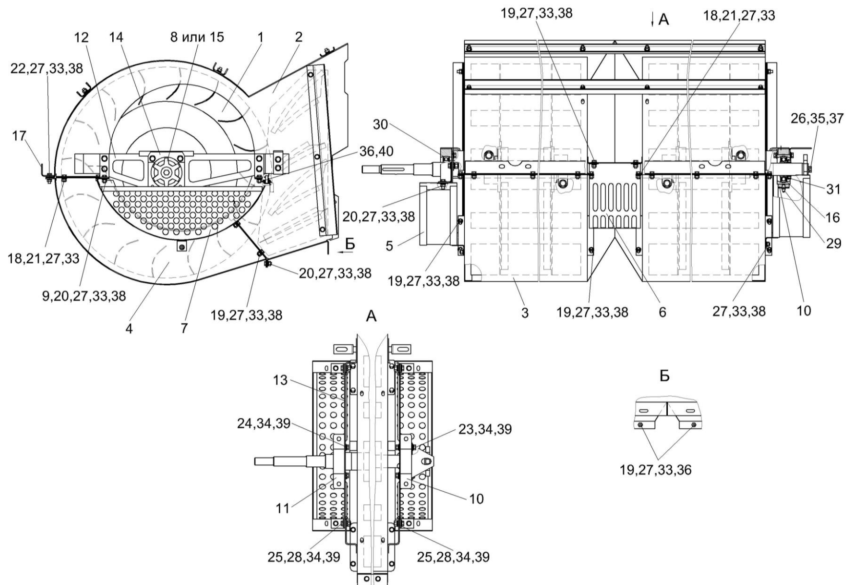
Рисунок 92 – Вентилятор КЗК-10-0217000
