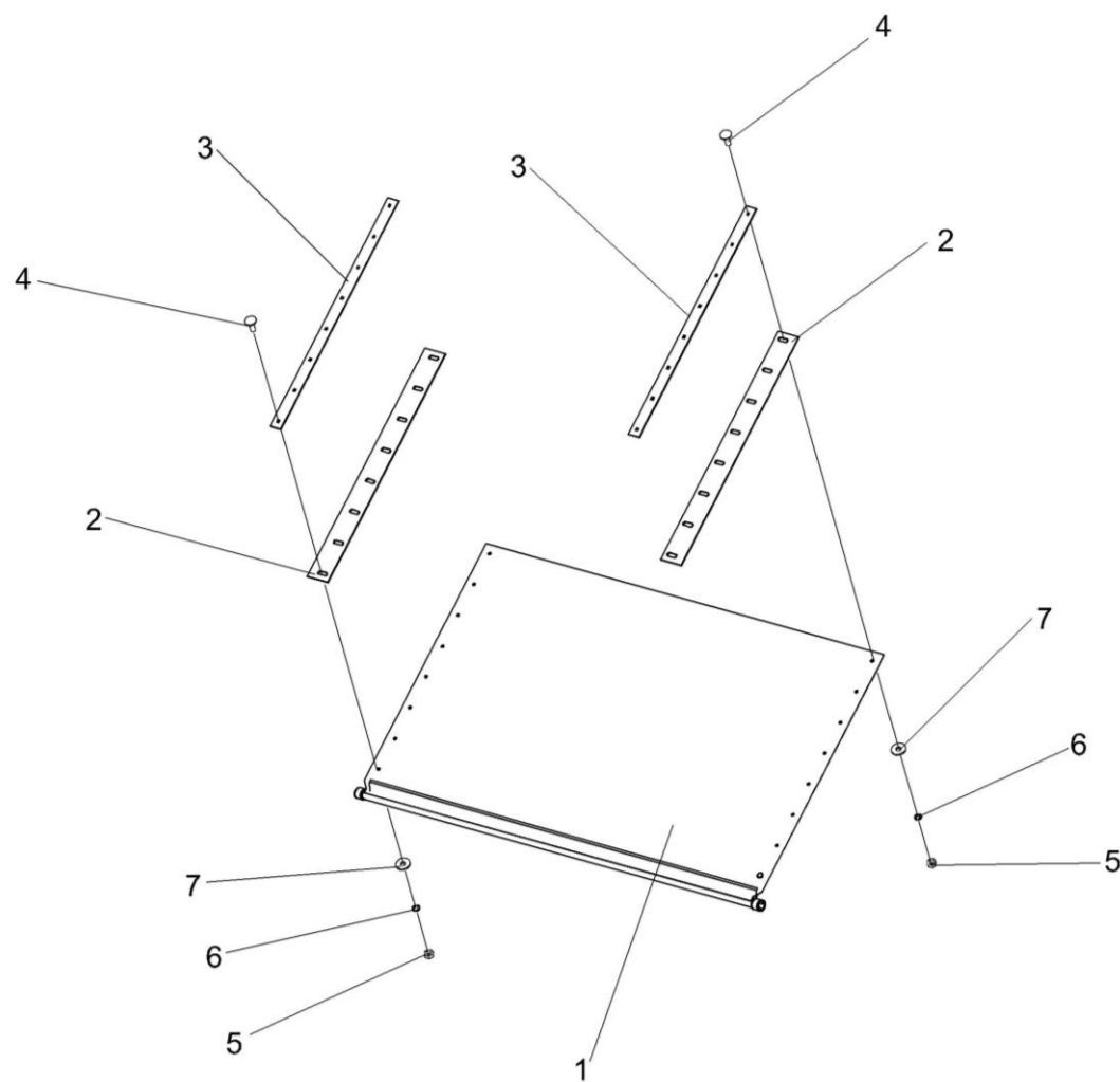
Рисунок 129 – Заслонка КЗК-10-0290160А
