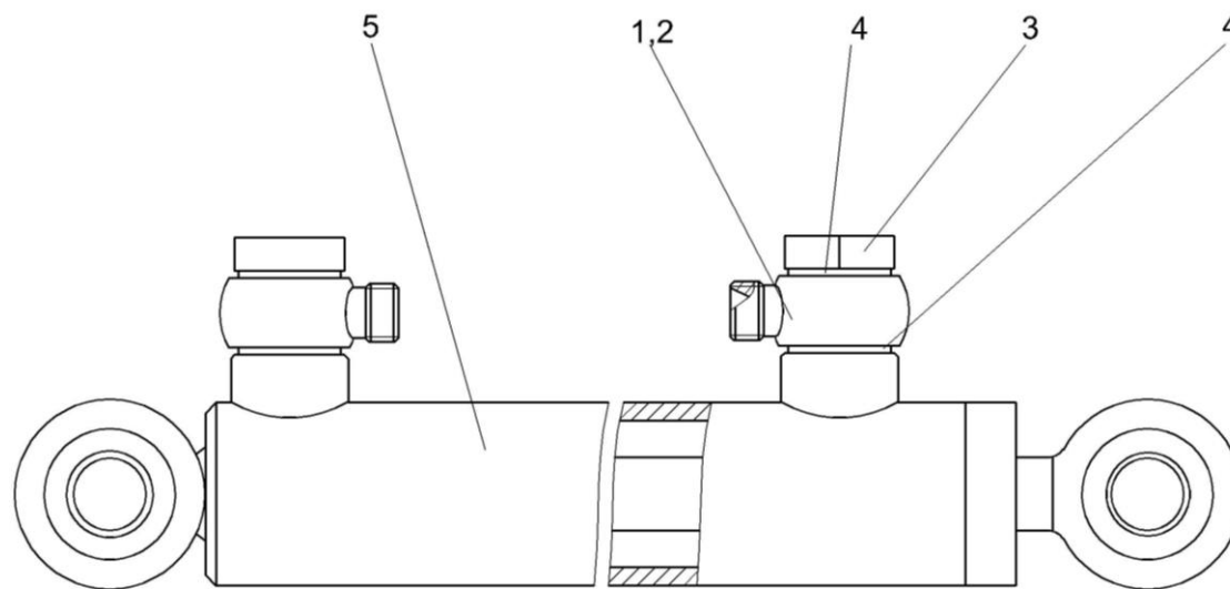
Рисунок 247 – Гидроцилиндр КЗК-12-0602700
