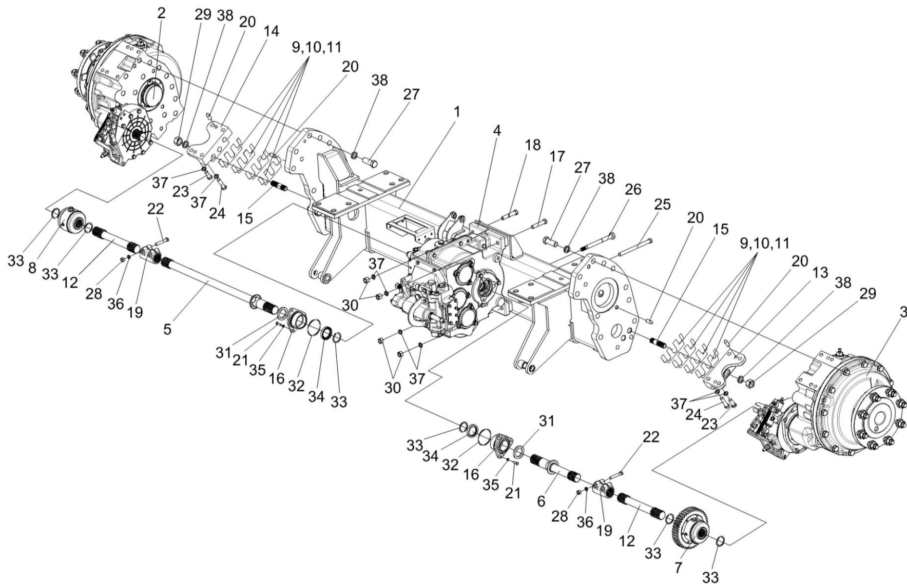
Рисунок 75 – Мост ведущий КЗК-12-0107300
