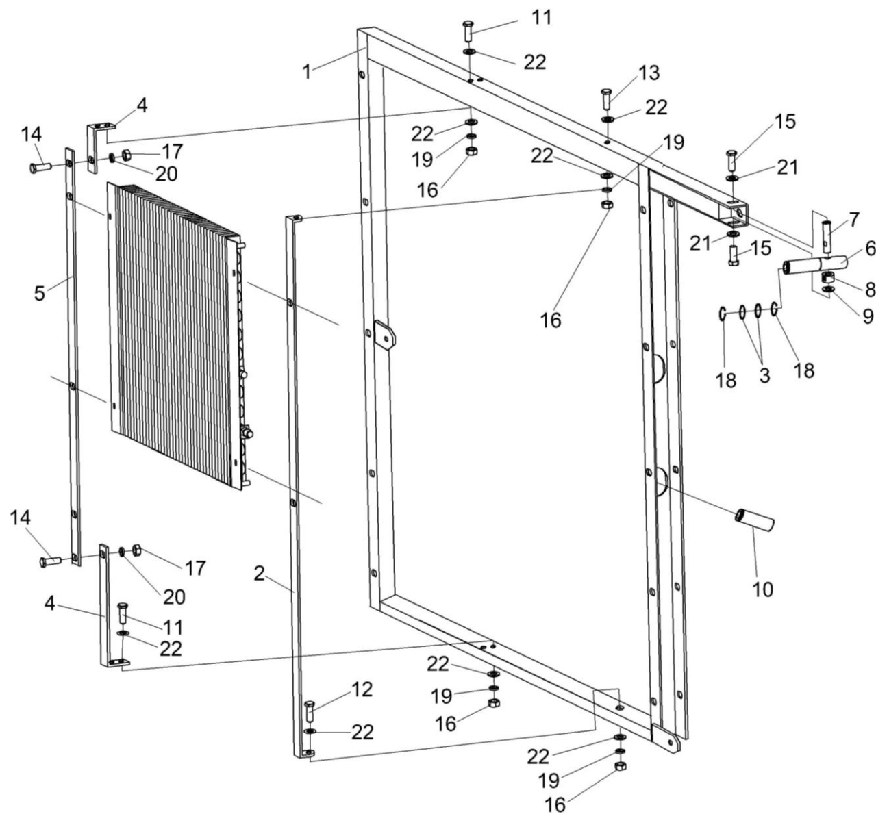
Рисунок 205 – Рама КЗК-12-3-0112080
