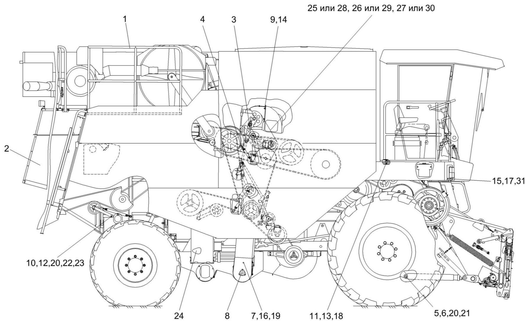
Рисунок 2 – Молотилка самоходная КЗК-12-0100000Б-10 (лист 2)
