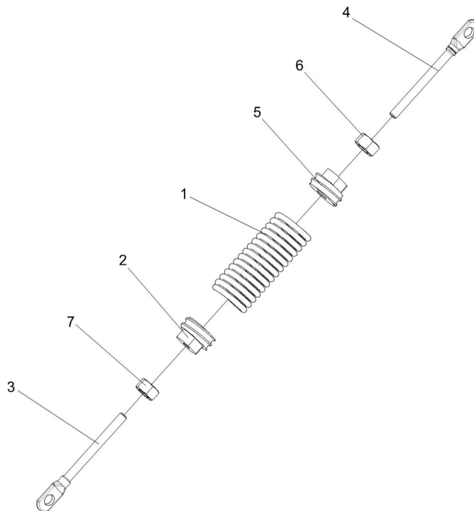
Рисунок 122 – Пружина КЗК-12-0221140А
