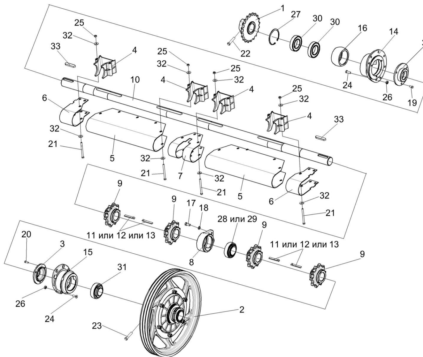
Рисунок 14 – Установка вала верхнего КЗС-12-1813000А
