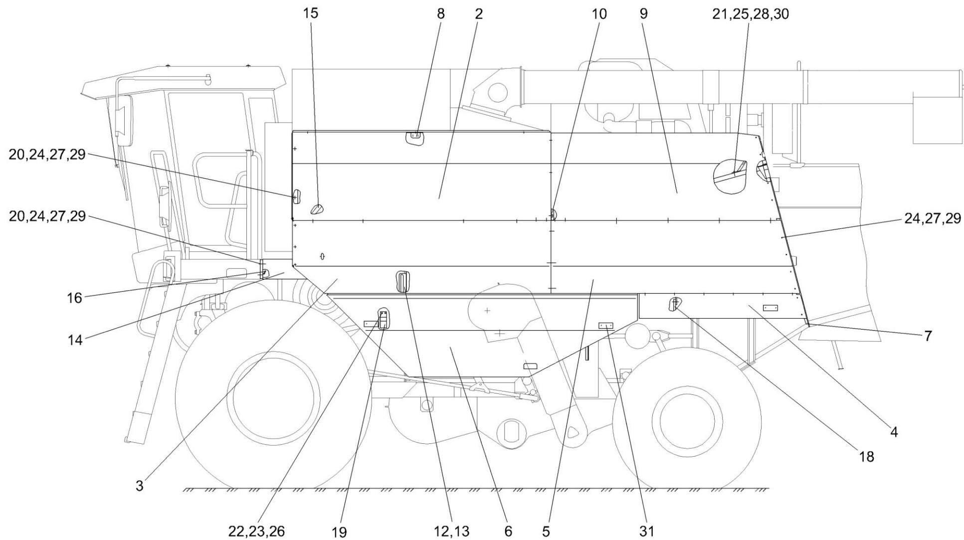
Рисунок 175 – Установка капотов и ограждения КЗК-12-0128000А (вид слева)
