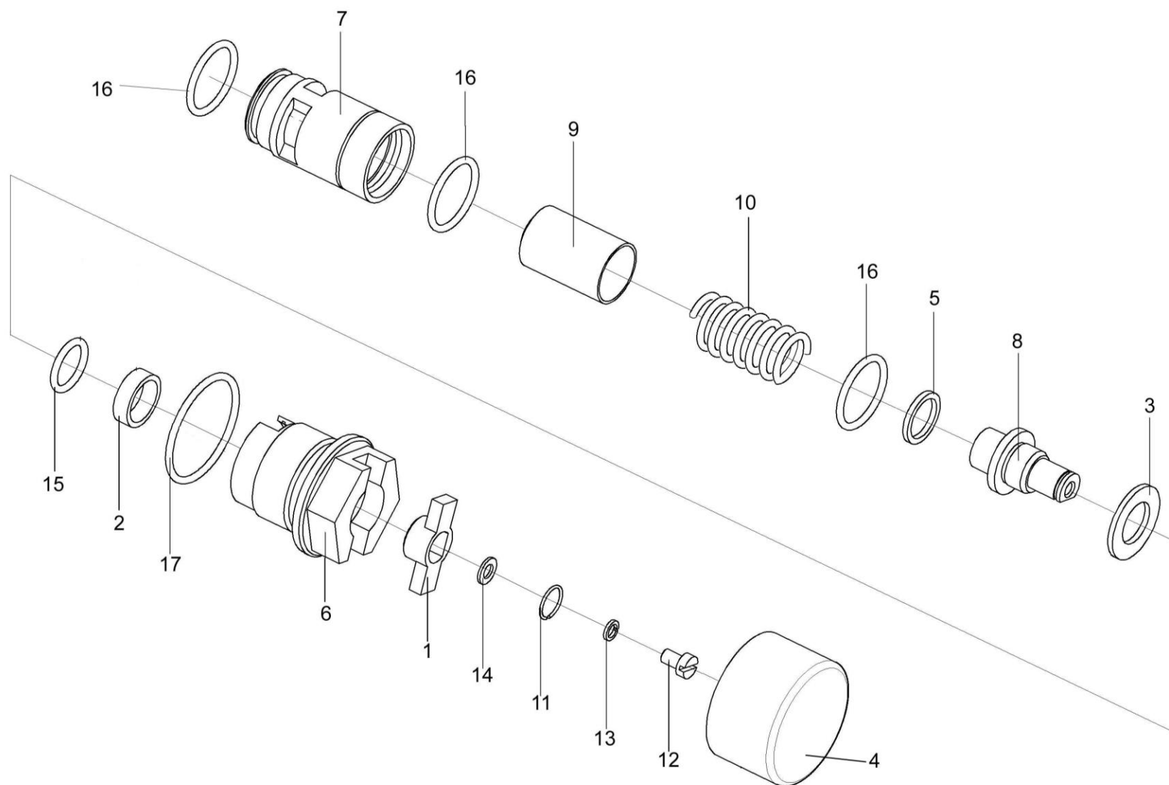
Рисунок 243 – Клапан-сигнализатор УЭС 0603660-01
