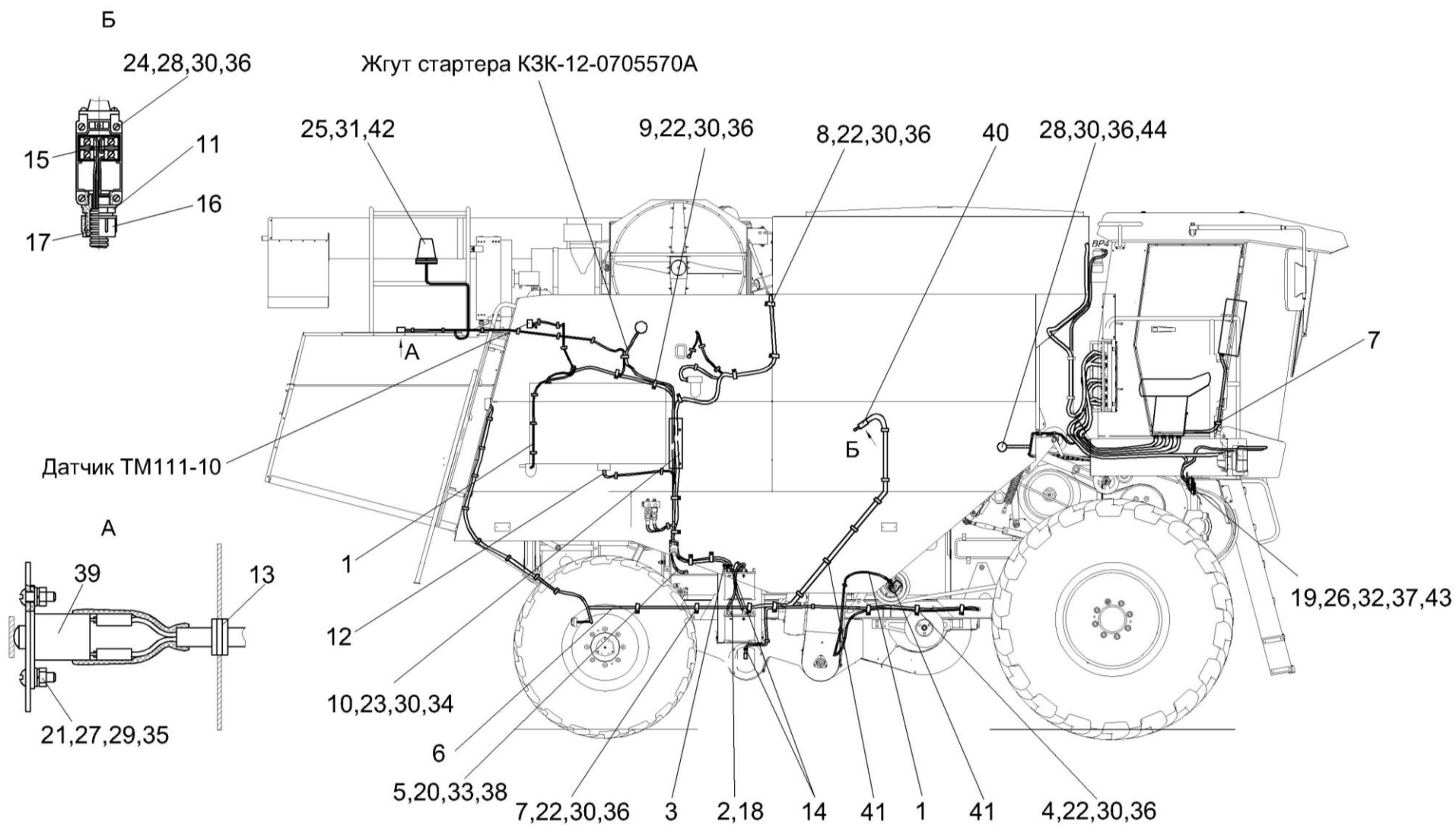
Рисунок 7 – Электрооборудование молотилки самоходной КЗК-12-0100000Б-10 (лист 2)
