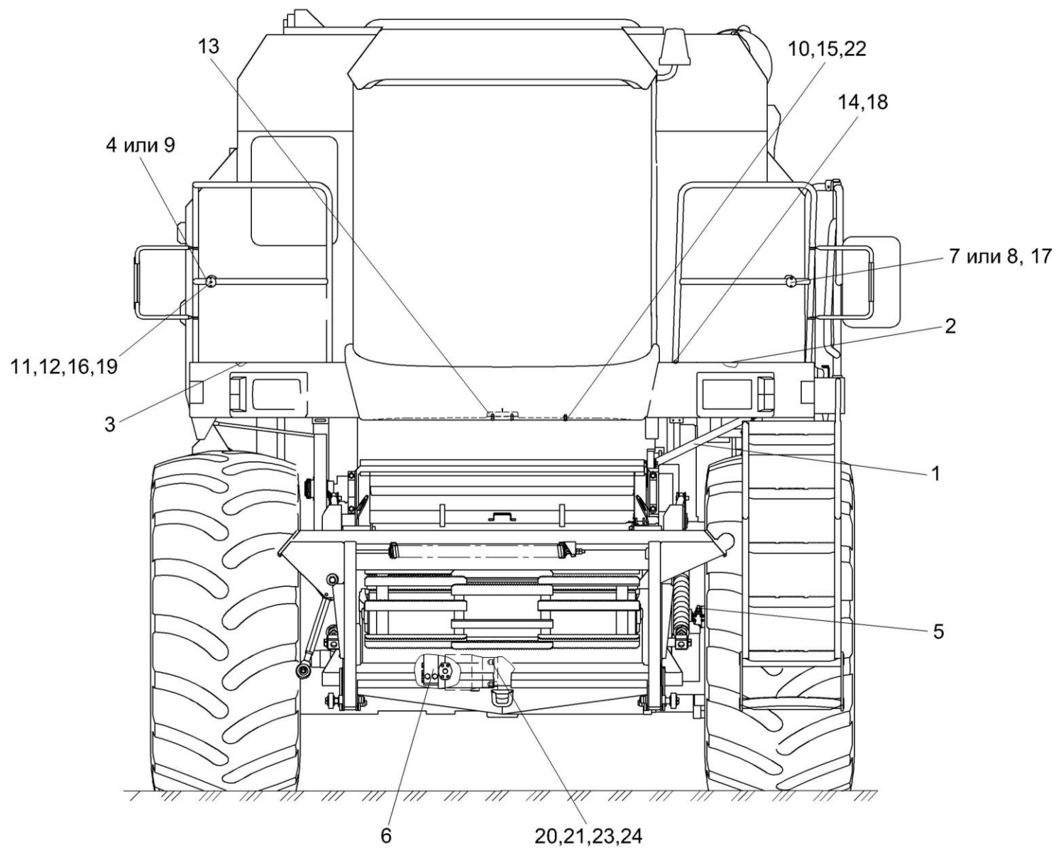
Рисунок 5 – Молотилка самоходная КЗК-12-0100000Б-10 (лист 5)
