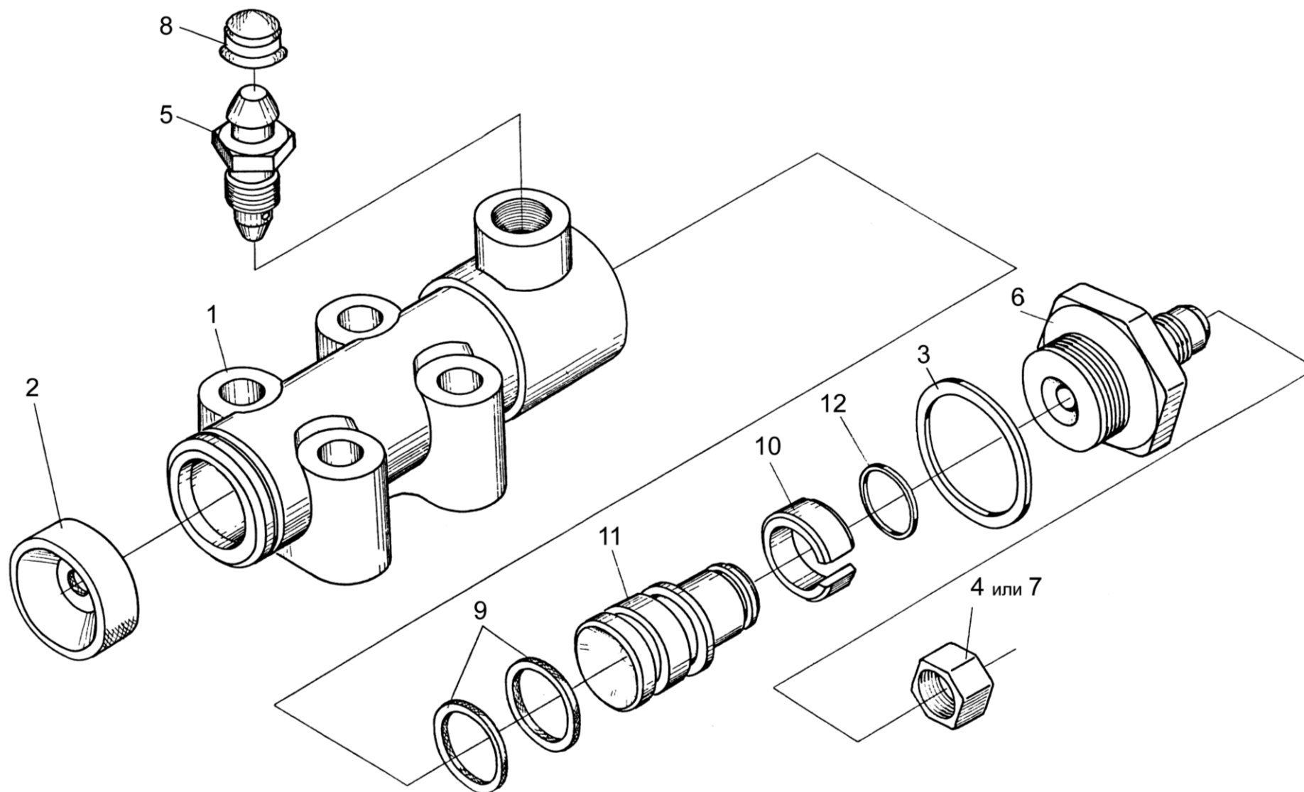
Рисунок 82 – Гидроцилиндр тормоза МК-23М.03.220А
