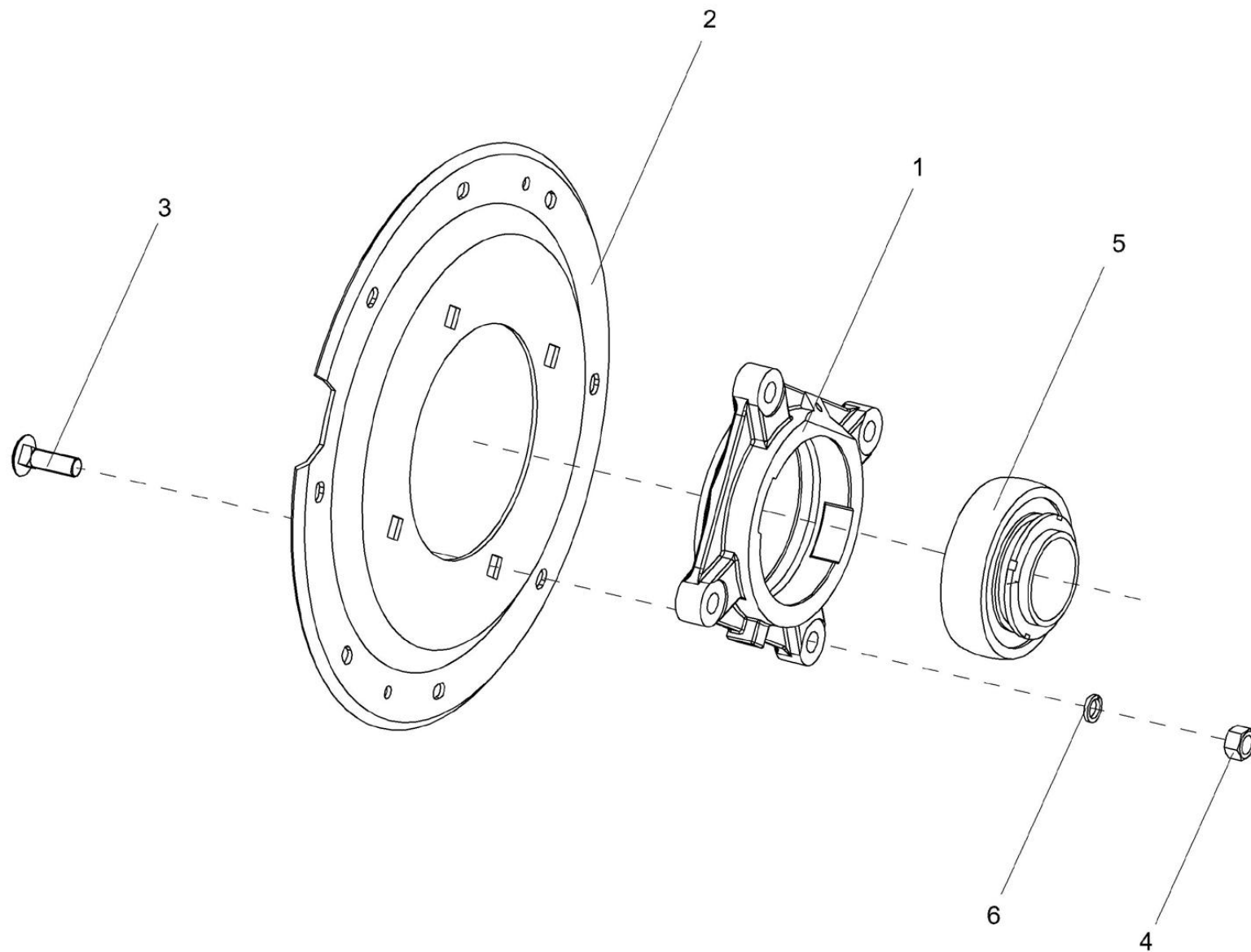
Рисунок 66 – Фланец КЗК-10-0102070
