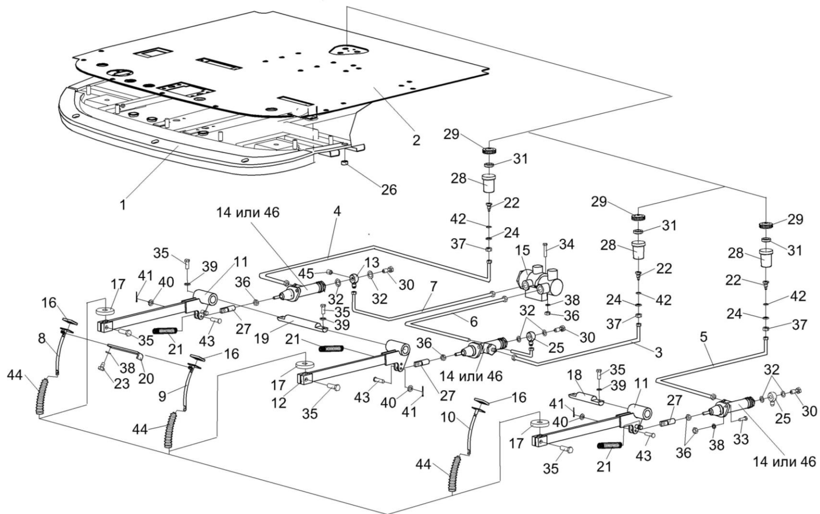
Рисунок 148 – Рычаги и трубопроводы площадки управления
