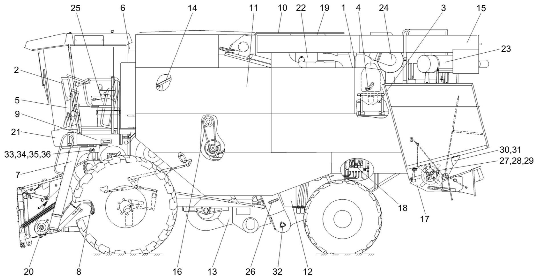
Рисунок 3 – Молотилка самоходная КЗК-12-0100000Б-10 (лист 3)
