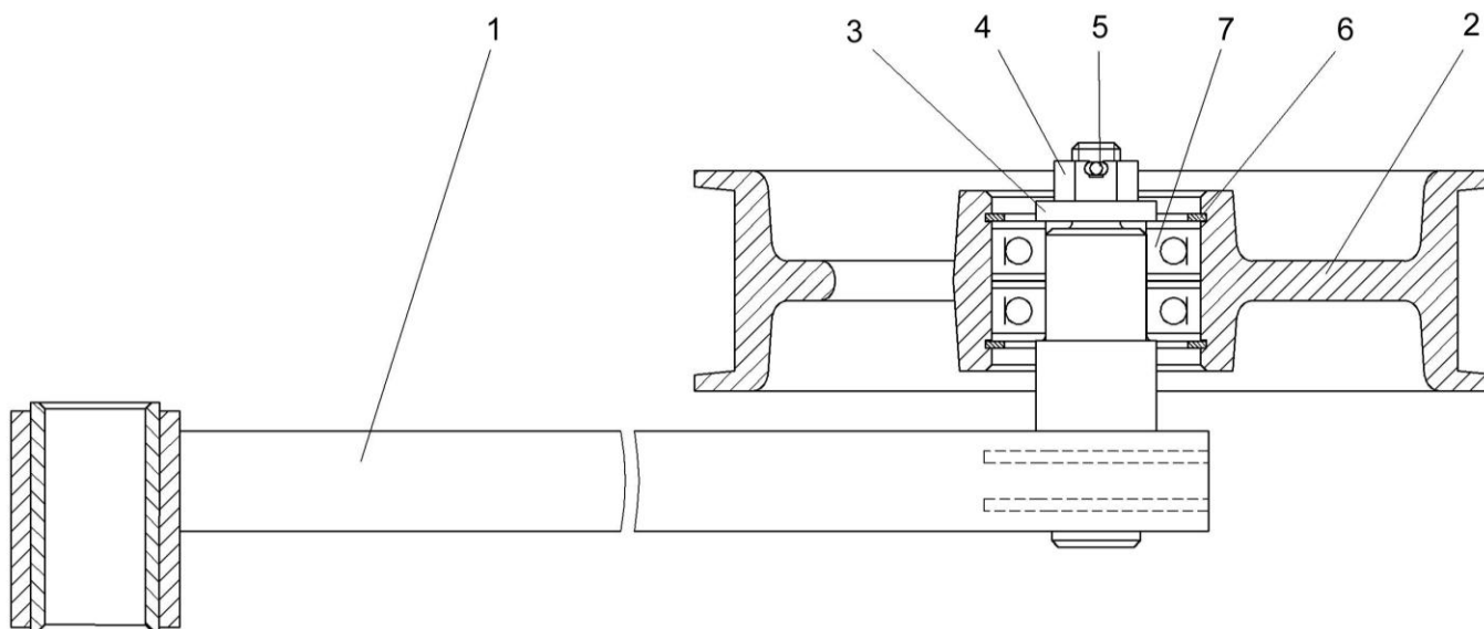
Рисунок 224 – Рычаг КЗК-10-0100620
