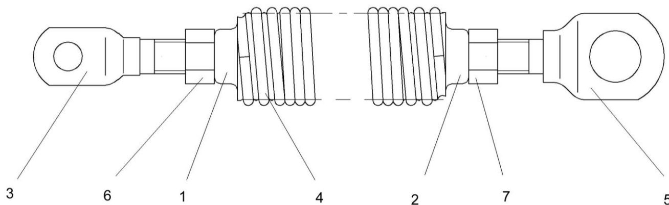
Рисунок 226 – Пружина КЗР-10-0100720А
