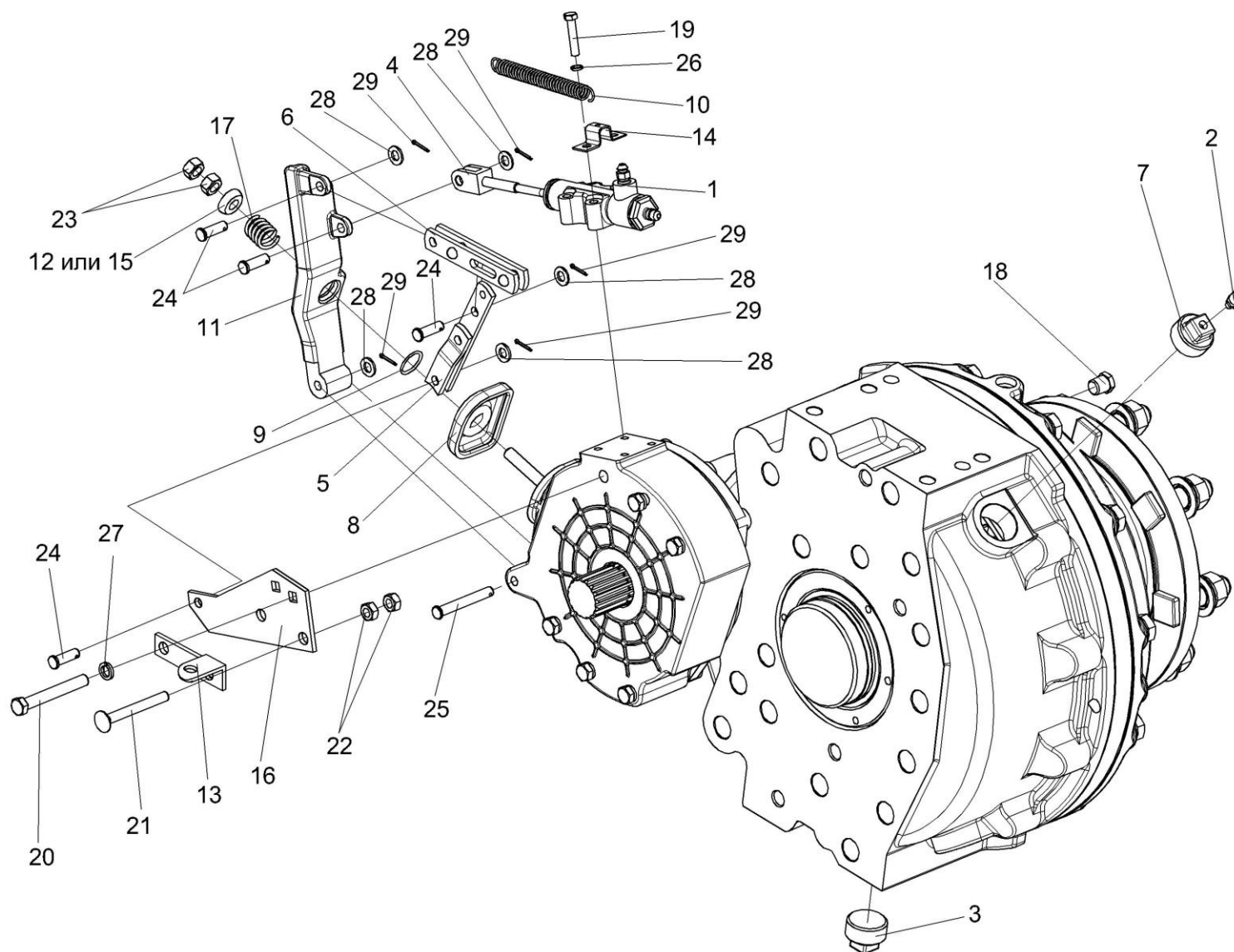
Рисунок 78 – Редуктор бортовой правый УЭС 0107070А-04 (лист 1)
