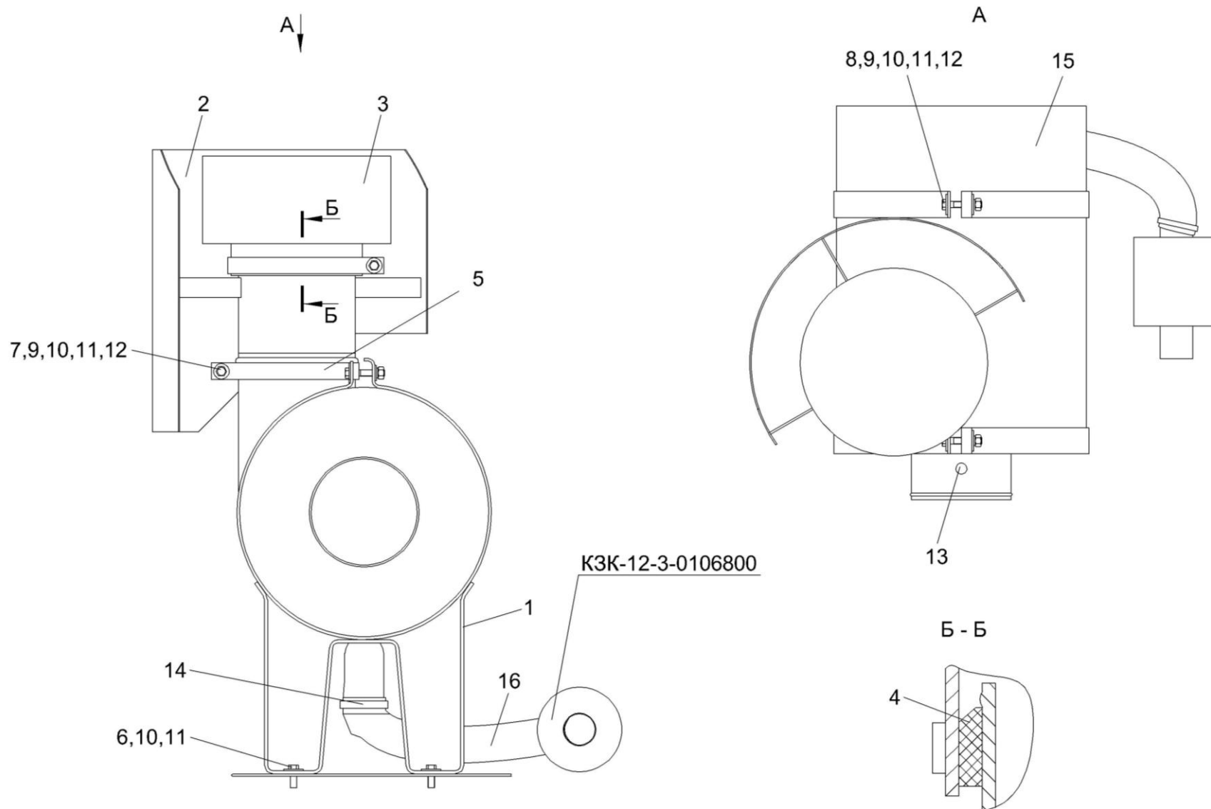
Рисунок 260 – Установка воздухоочистителя G150092 K3K-12-3-0106760
