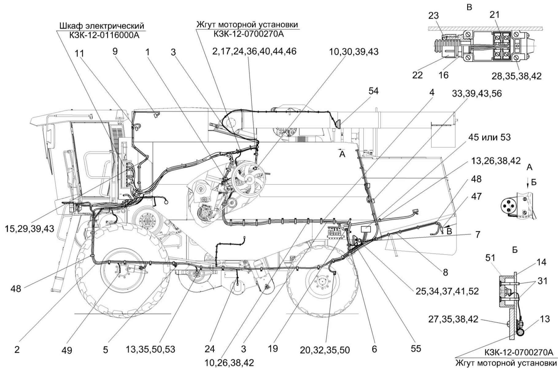
Рисунок 6 – Электрооборудование молотилки самоходной КЗК-12-0100000Б-10 (лист 1)
